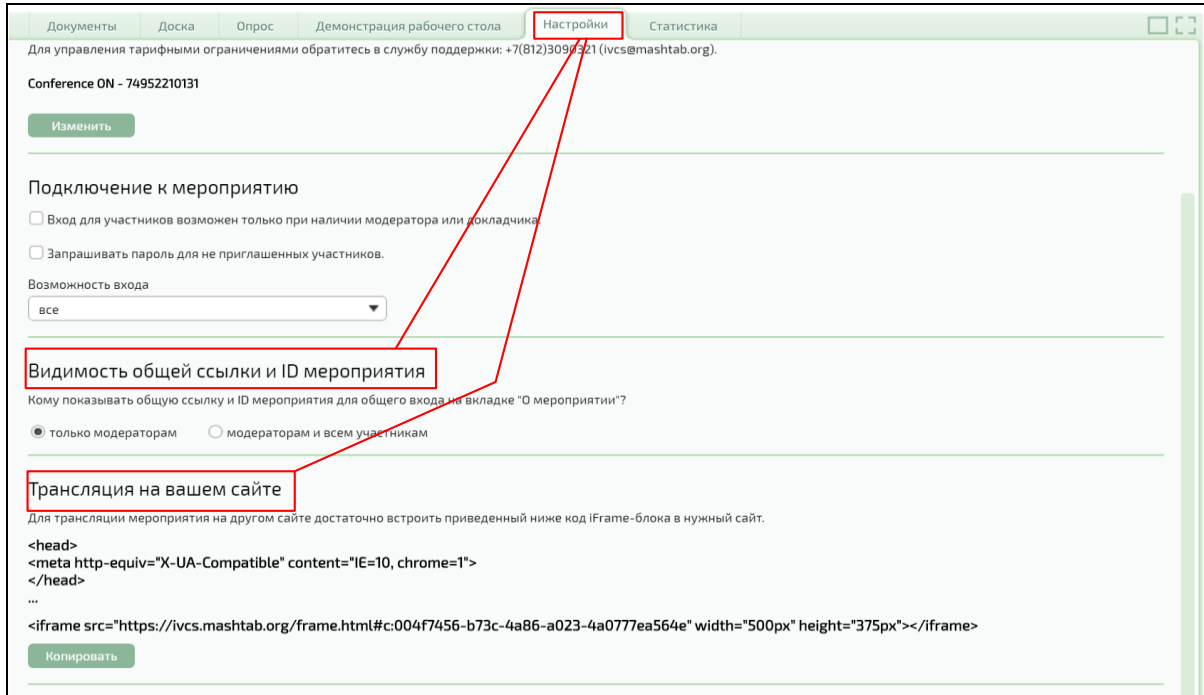
Рис. 141 – Получение кода для встраивания в сторонний сайт
