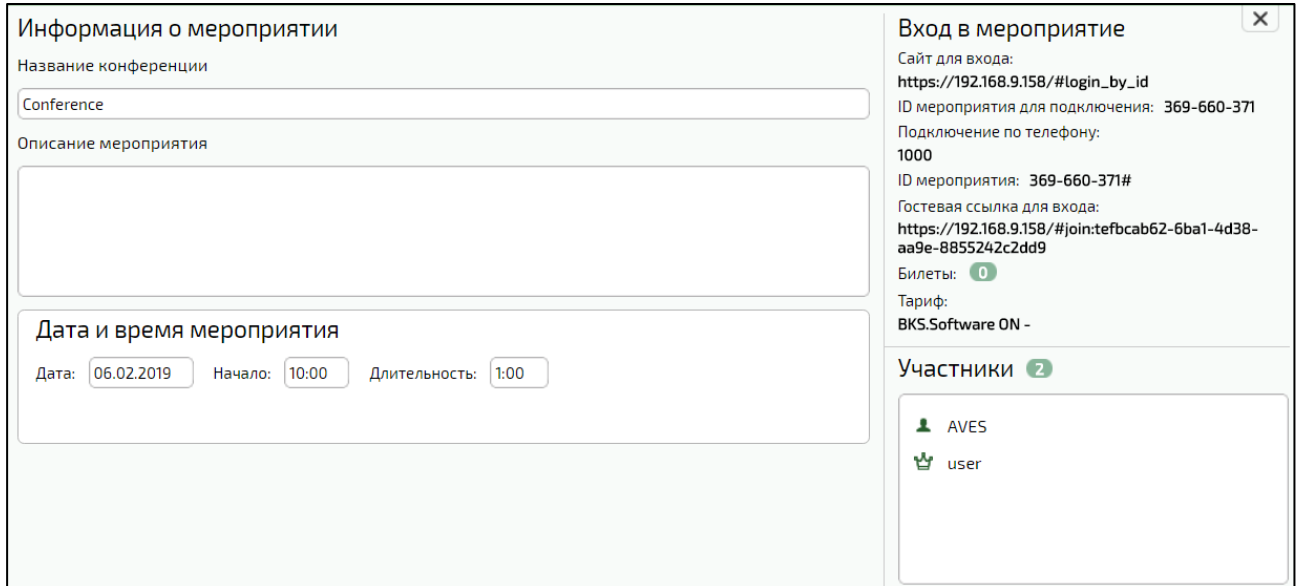
Рис. 44 – Просмотр настроек мероприятия
